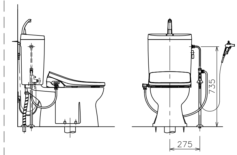
右側壁給水時の接続位置
