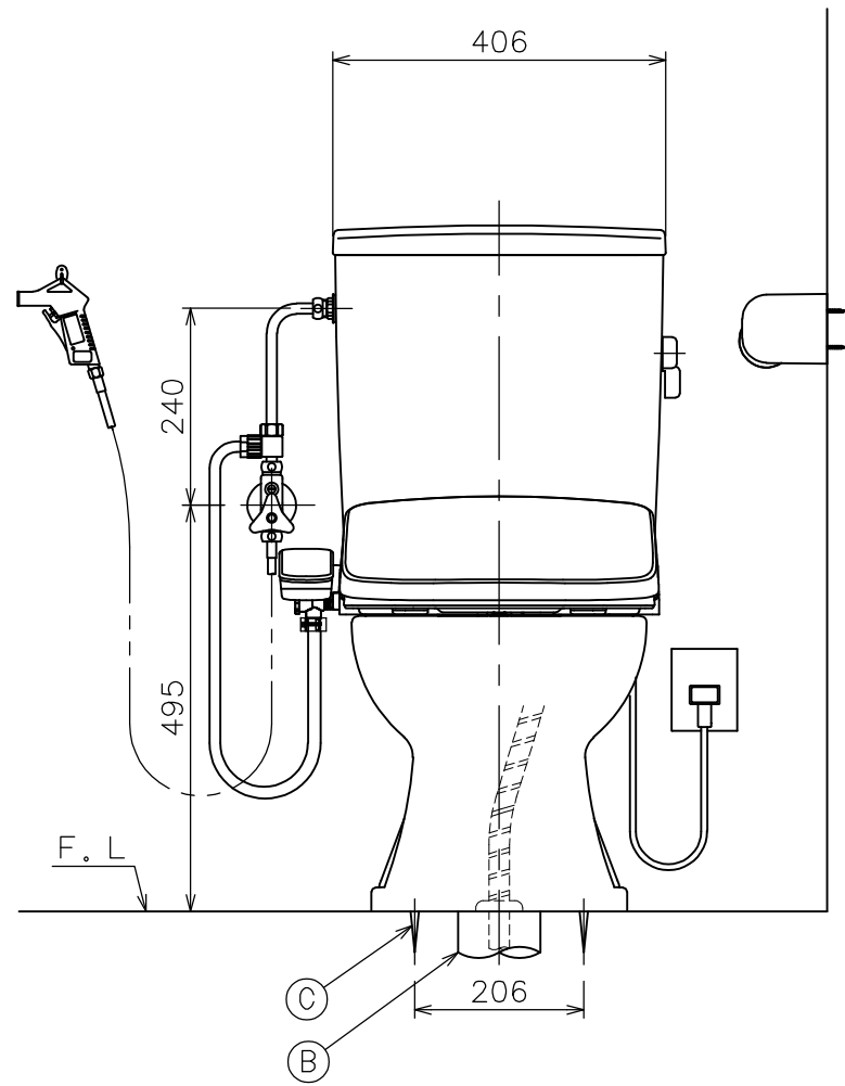
左側壁給水時の接続位置（標準）
