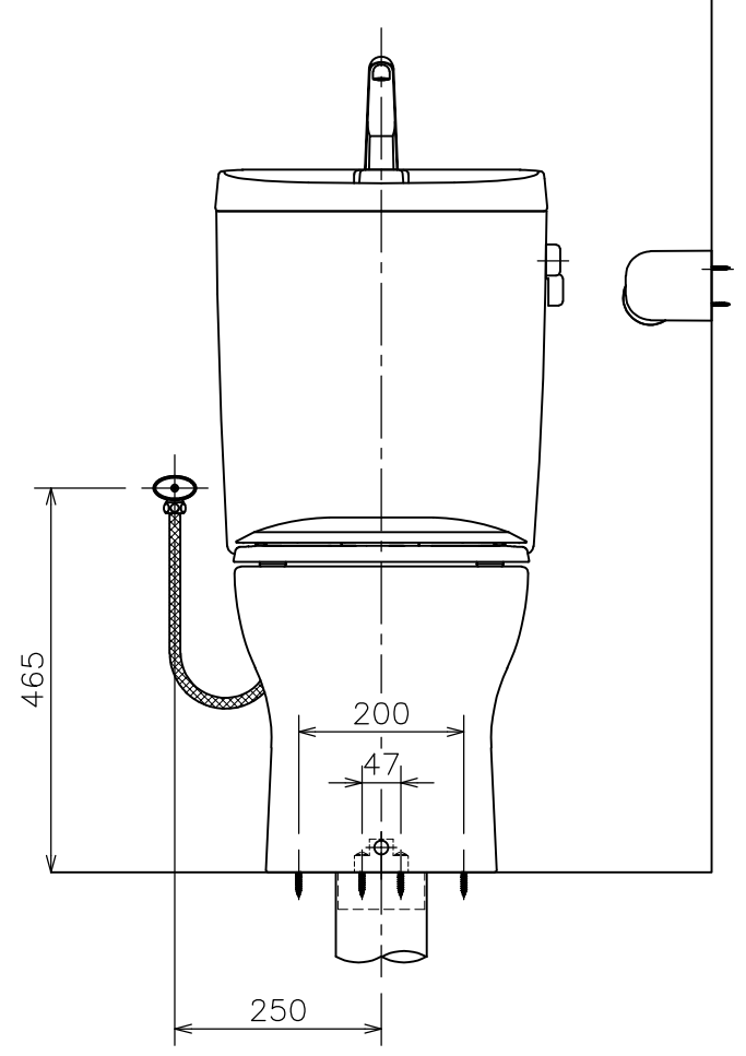
左側壁給水時の接続位置(標準)
