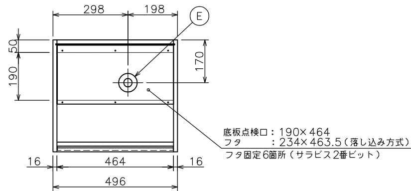
給・排水取り合い図
