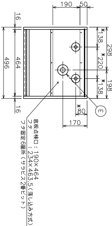
給・排水取り合い図
