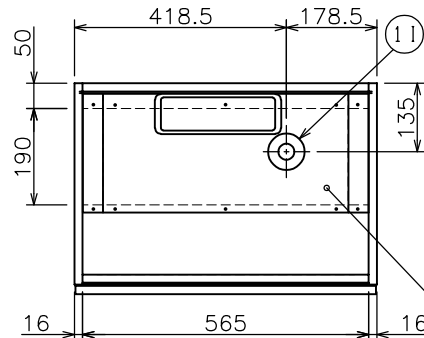
排水取り合い図
