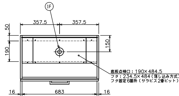
排水取り合い図
