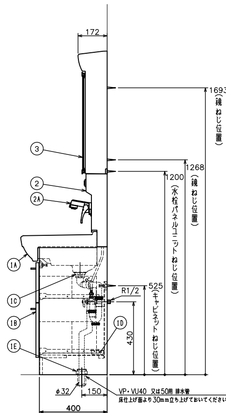
排水取り合い図
